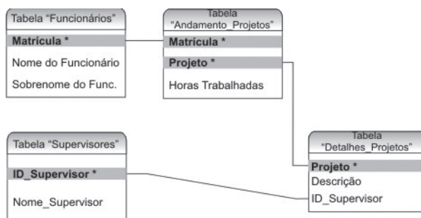
Figura 1.15: O banco de dados usado para o nosso exemplo, respeita agora as três Formas Normais. Veja como cada tabela está relacionada com a(s) outra(s).
