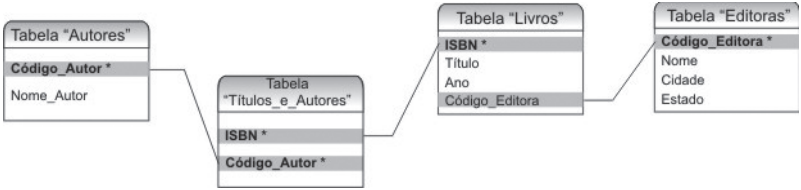
Figura 1.14: Representação esquemática de um relacionamento muitos-para-muitos.
